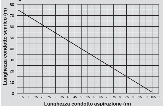
Lunghezza massima tubi Ø 80 mm - 25 IS
