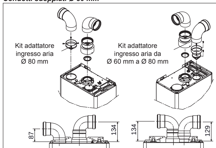
Lunghezza massima tubi Ø 80 mm - 25 IS
